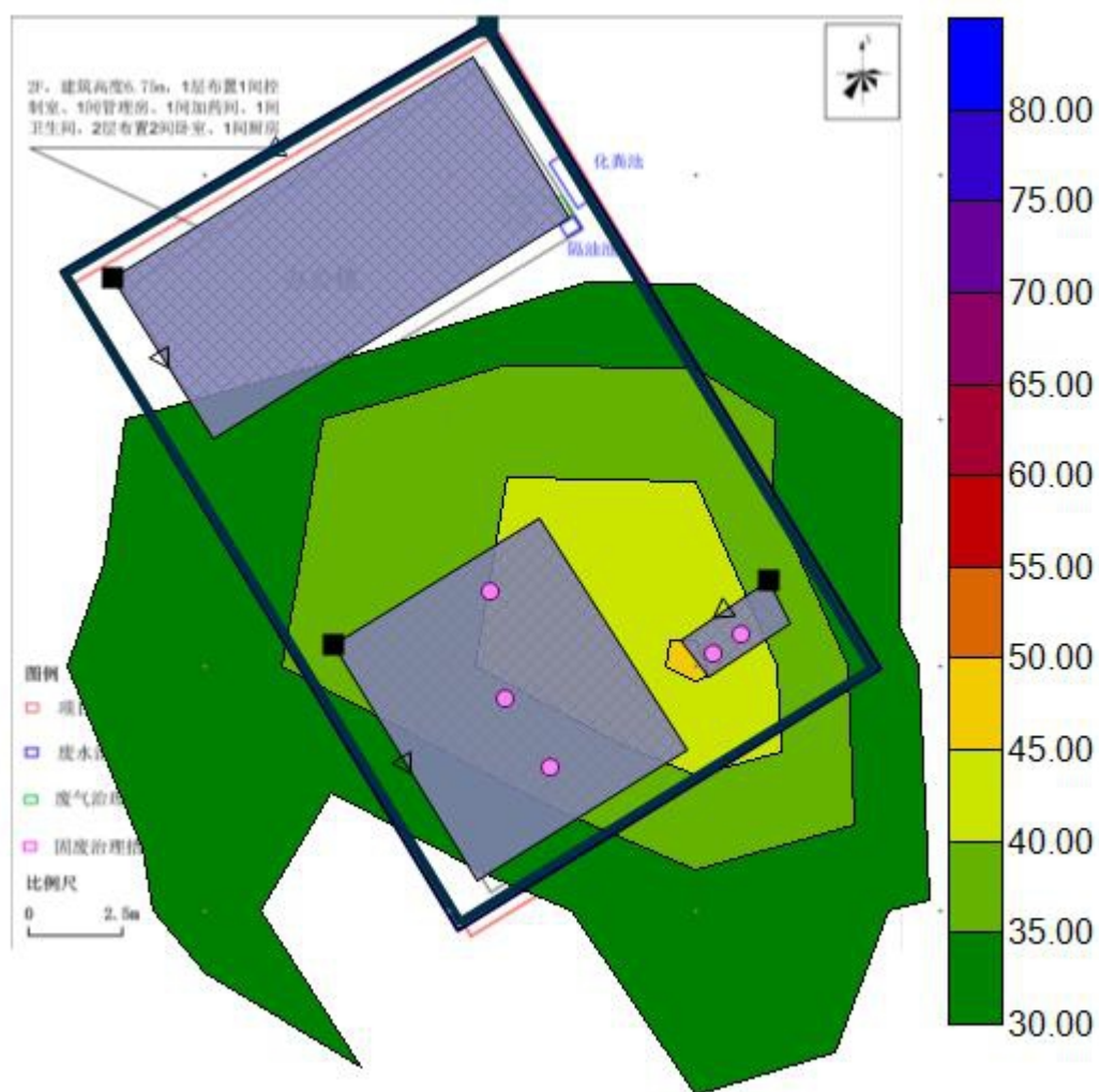
图 4-4 乌东德老集镇水厂噪声等声值线图（昼、夜）
