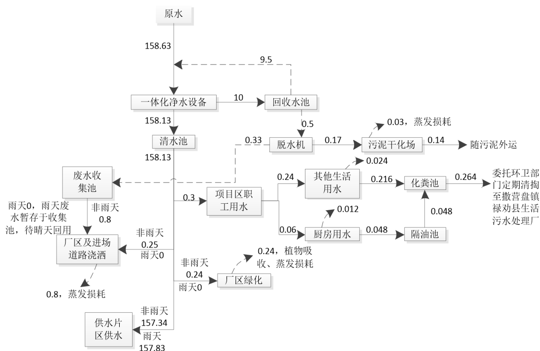
图 2-6 撒营盘镇德嘎村水厂水平衡图 单位: m 3 /d
