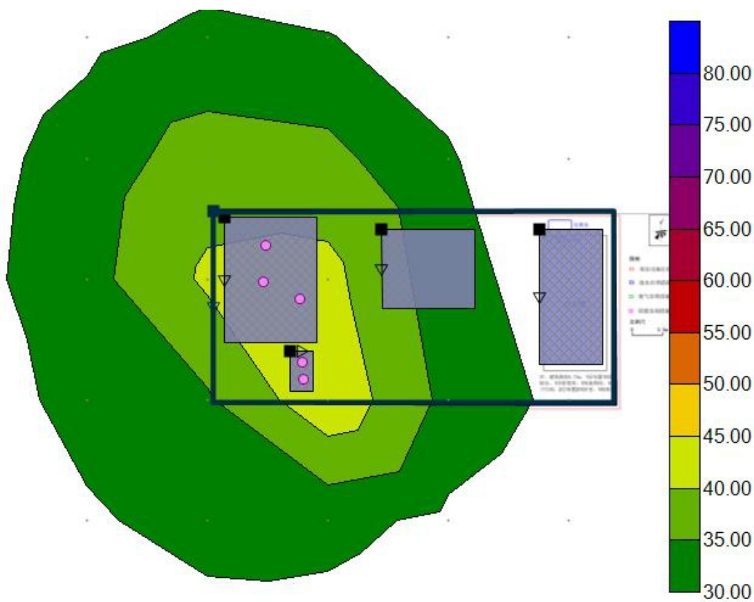
图 4-6 汤郎乡水厂运营期噪声等声值线图（昼、夜）
