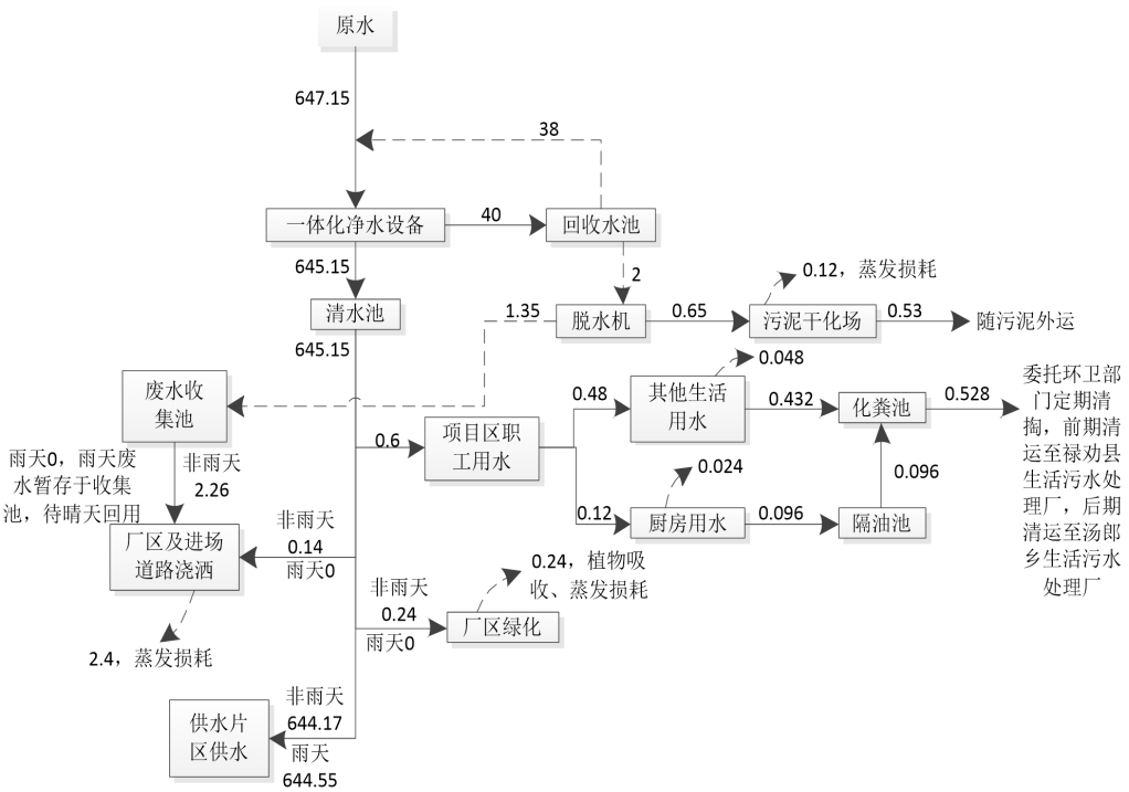
图 2-5 汤郎乡水厂水平衡图 单位：m³/d
