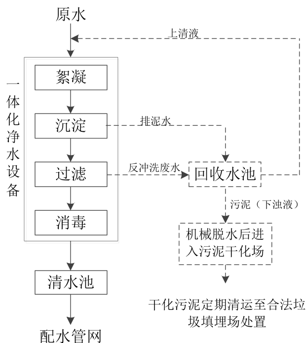
图 2-9 运营期工艺流程及产污节点图
