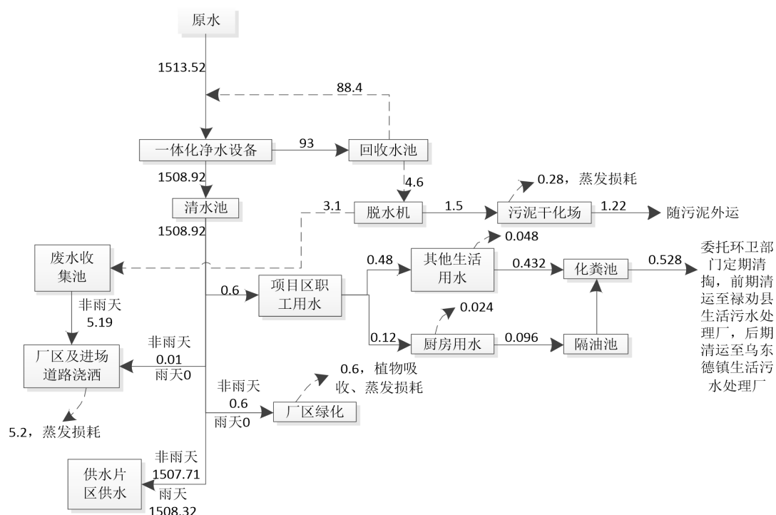
图 2-2 乌东德新集镇水厂水平衡图 单位: m³/d
