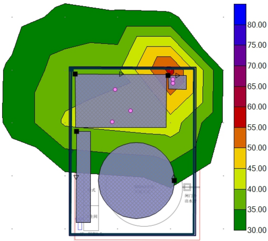
图 4-2 皎平渡发展片区水厂运营期噪声等声值线图（昼、夜）
