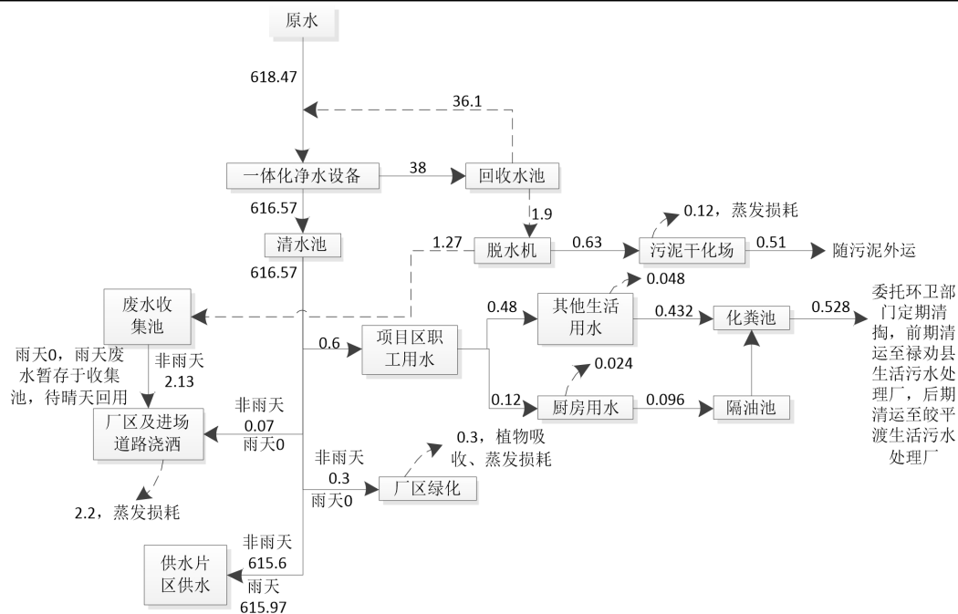
图 2-1 皎平渡发展片区水厂水平衡图 单位: \text{m}^3/\text{d}
