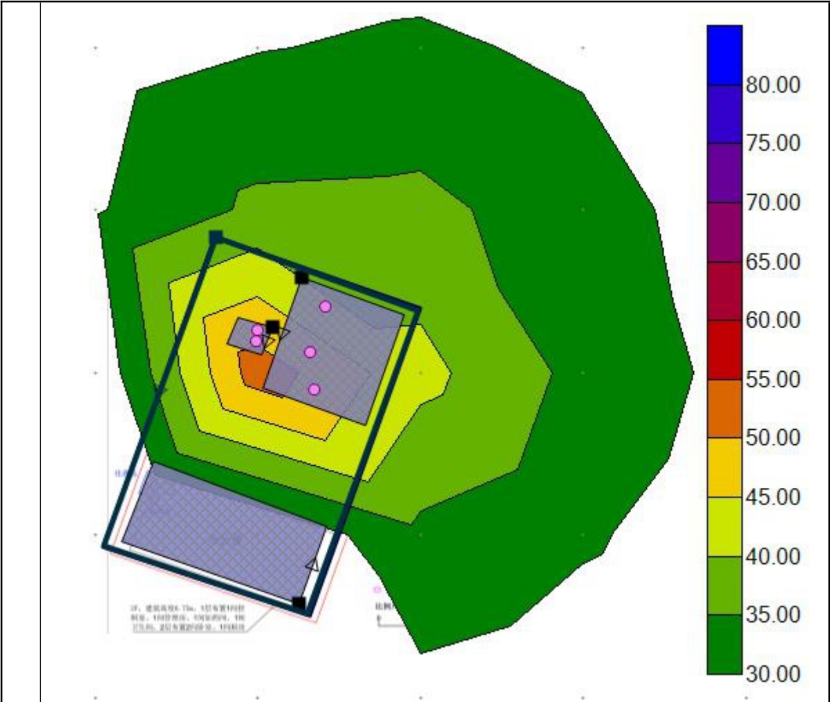
图 4-5 团街镇治安村水厂运营期噪声等声值线图（昼、夜）
