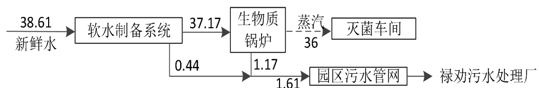
图 2-1 项目水平衡图 (t/d)
