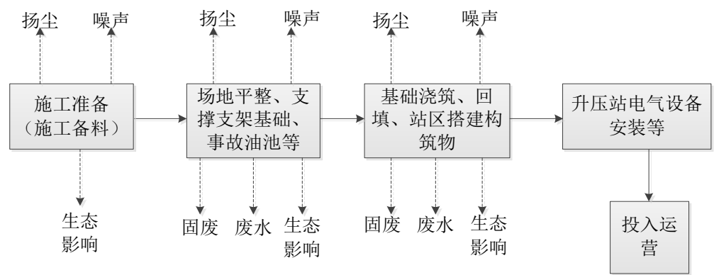
图4-2 升压站施工工艺流程及产污环节图
