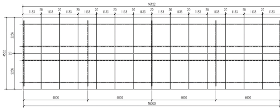
图 2-1 晶体硅单支架方阵面组件纵向排列
