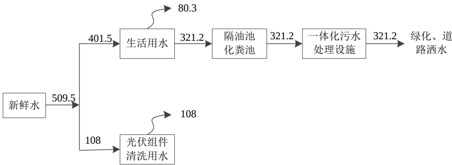
图 2-1 项目水量平衡图 m 3 /a
