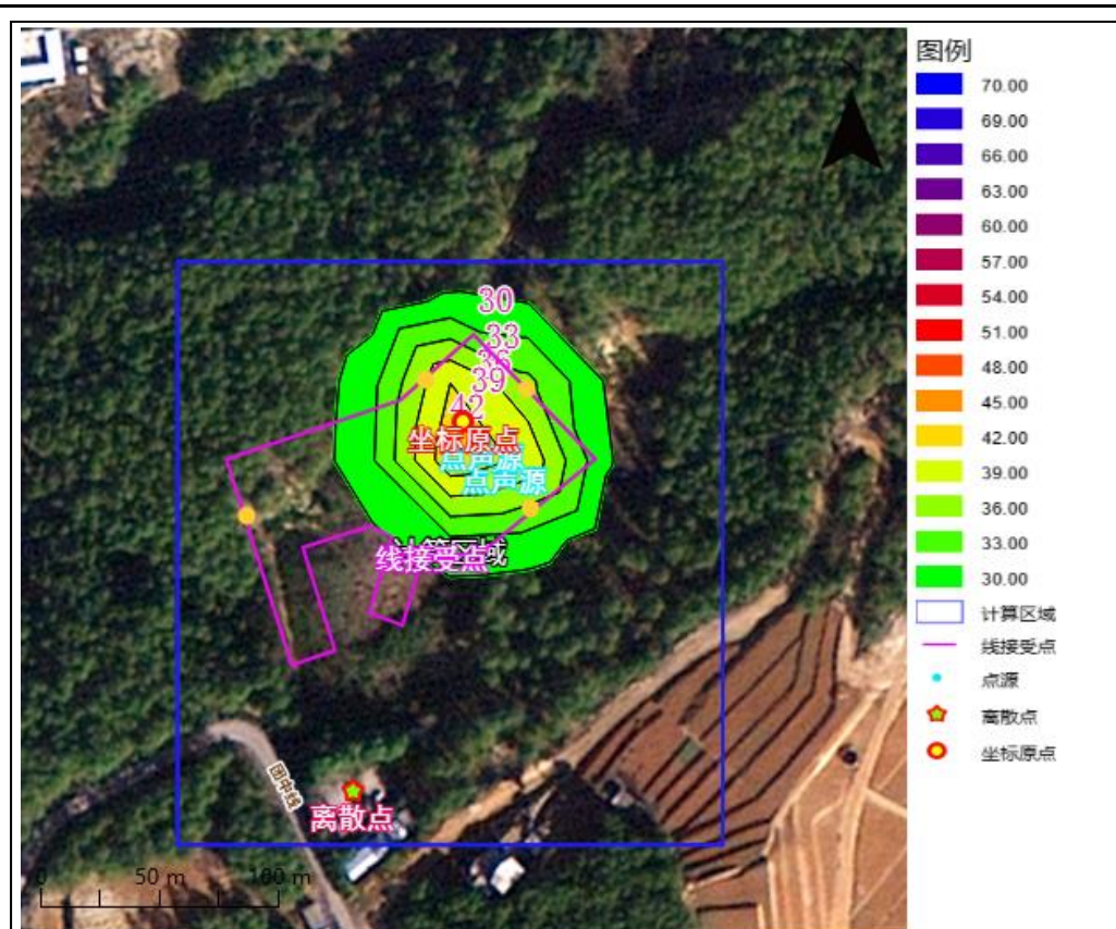
图 4-1 项目运营期等声级线图 单位：dB (A)
