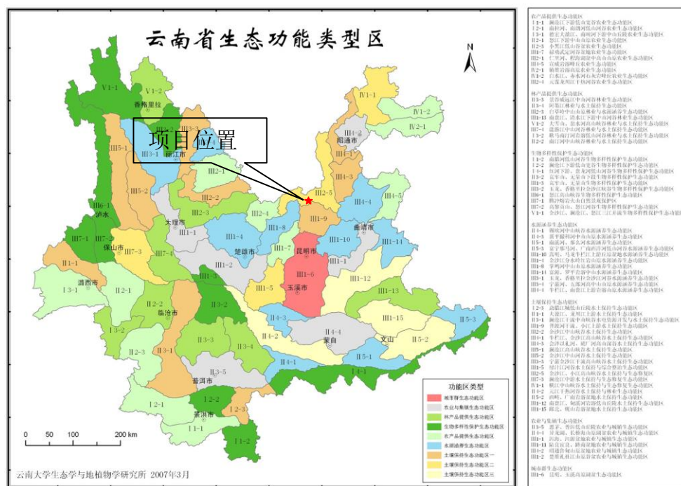
图 3-2 云南省生态功能区划图
