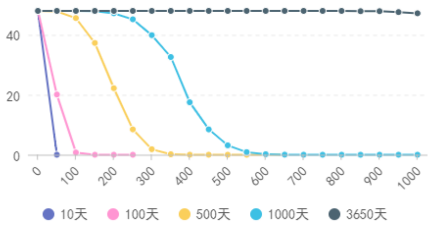
图5.3-8 氨氮随距离和时间变化曲线
