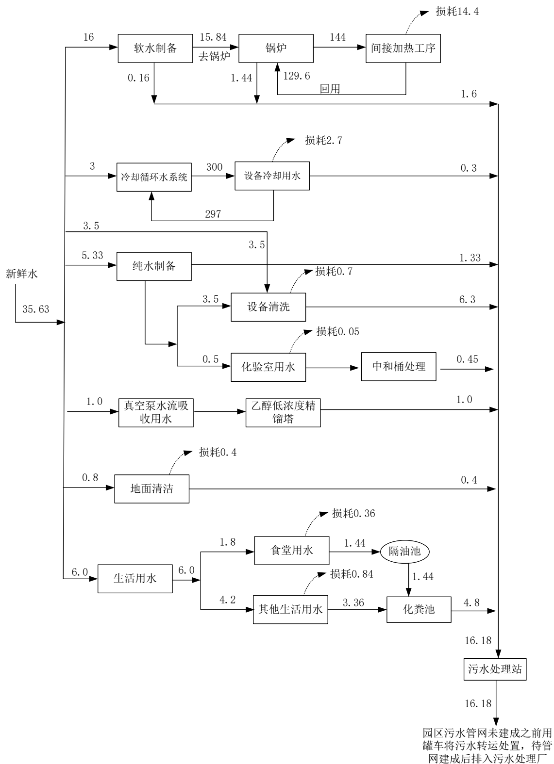
图 2.2-9 项目雨天水平衡图 单位: \text{m}^3/\text{d}
