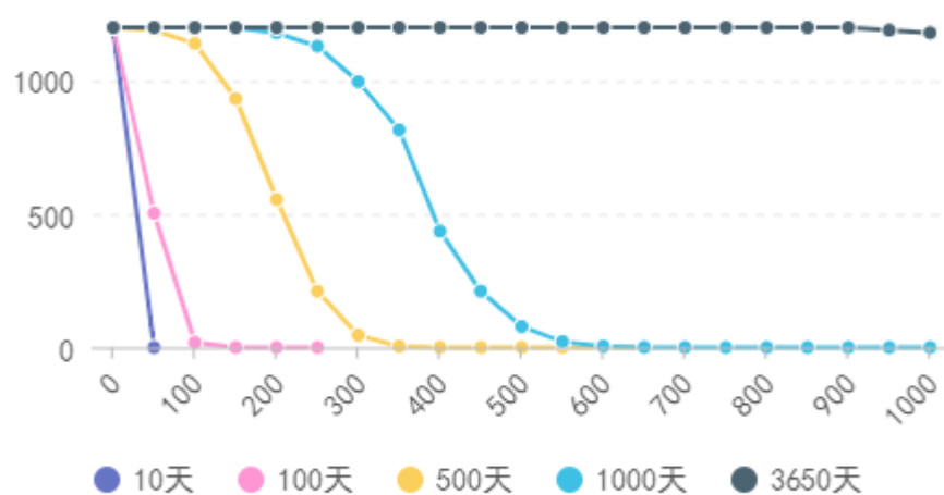
图5.3-7 COD随距离和时间变化曲线
