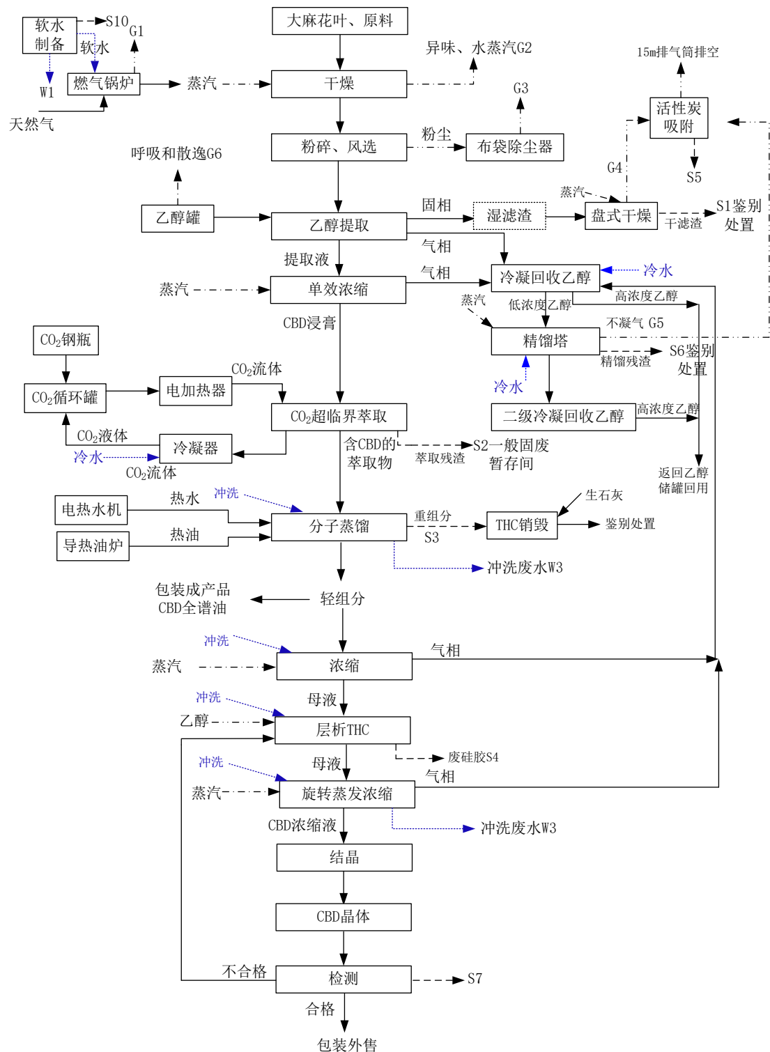
图 2.2-2 项目生产工艺流程及产污节点图
