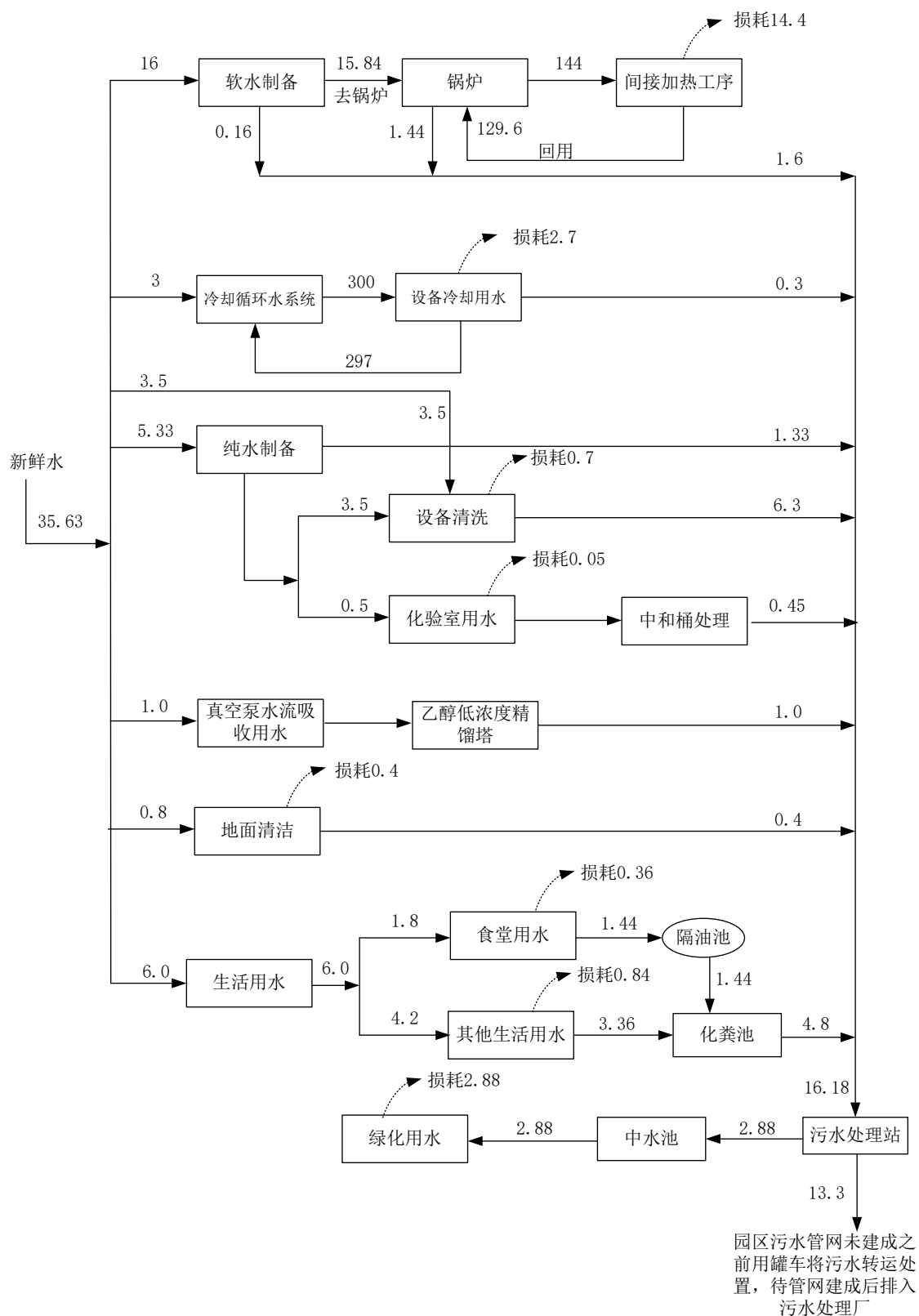
图 2.2-8 项目区晴天水平衡图 单位: \text{m}^3/\text{d}
