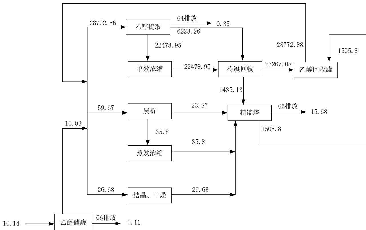
图 2.2-5 项目乙醇平衡图 单位：t/a
