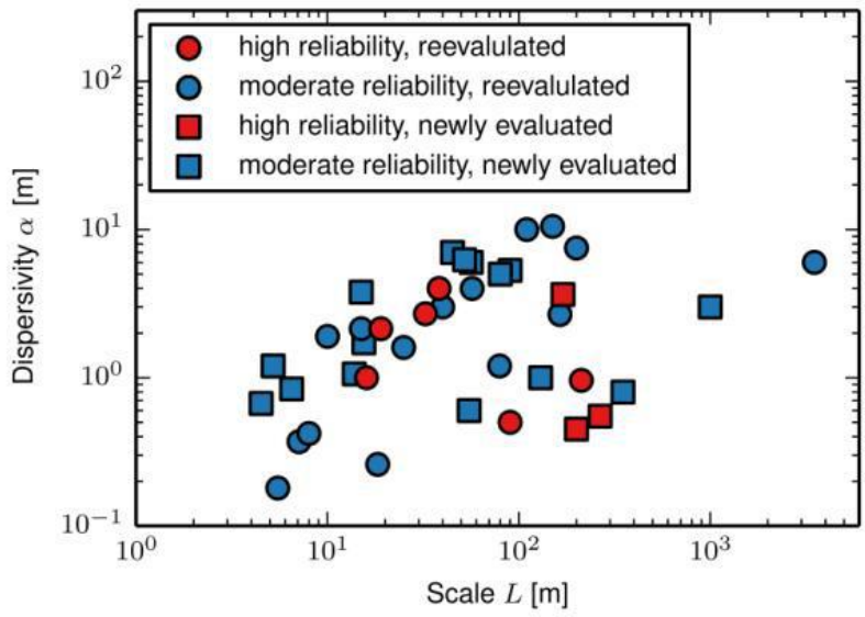
图 5.3-2 弥散度与区域尺度关系图
