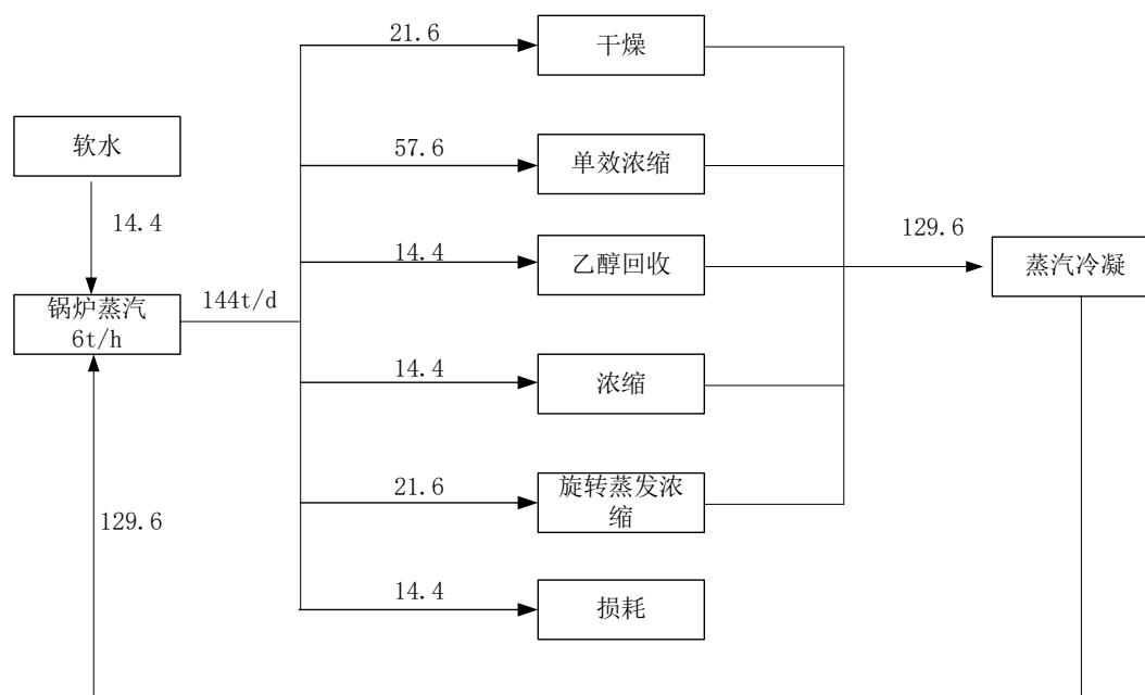
图 2.2-6 项目蒸汽平衡图 单位: t/d
