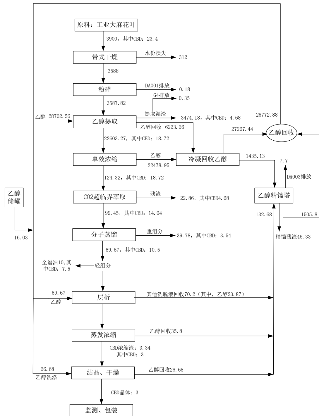
图 2.2-4 项目物料平衡图 单位: t/a
