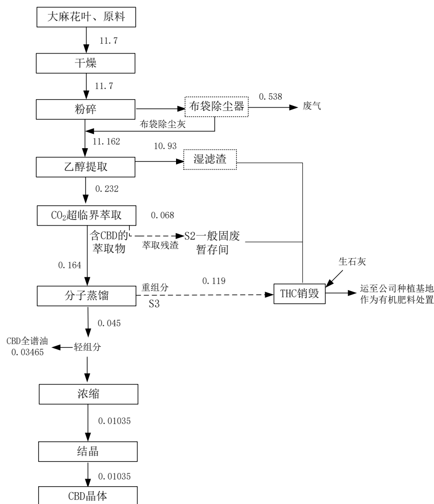
图 2.2-7 项目 THC 平衡图 单位: t/d
